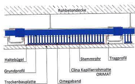
Deckenschnitt
